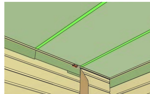
11. Leikkaa ylimääräiset ilman/höyrynsulut rimojen alareunaa vasten pois.
