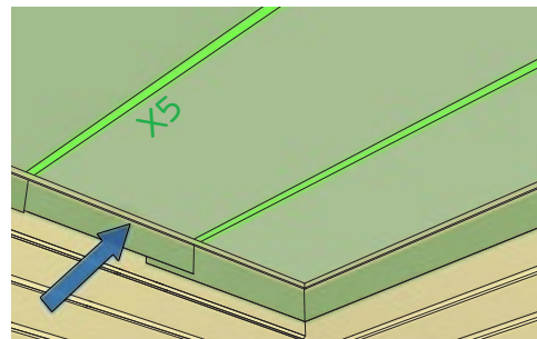
10. Varmista ilman/höyrynsulun ja seinän tiiviyys seiniin kiinnitettävällä rimalla.
